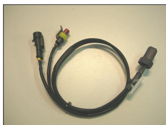
Cavo iniettore Tipo E3 Delphi (4 pin) n° 20584346 COD.:555-90-2
